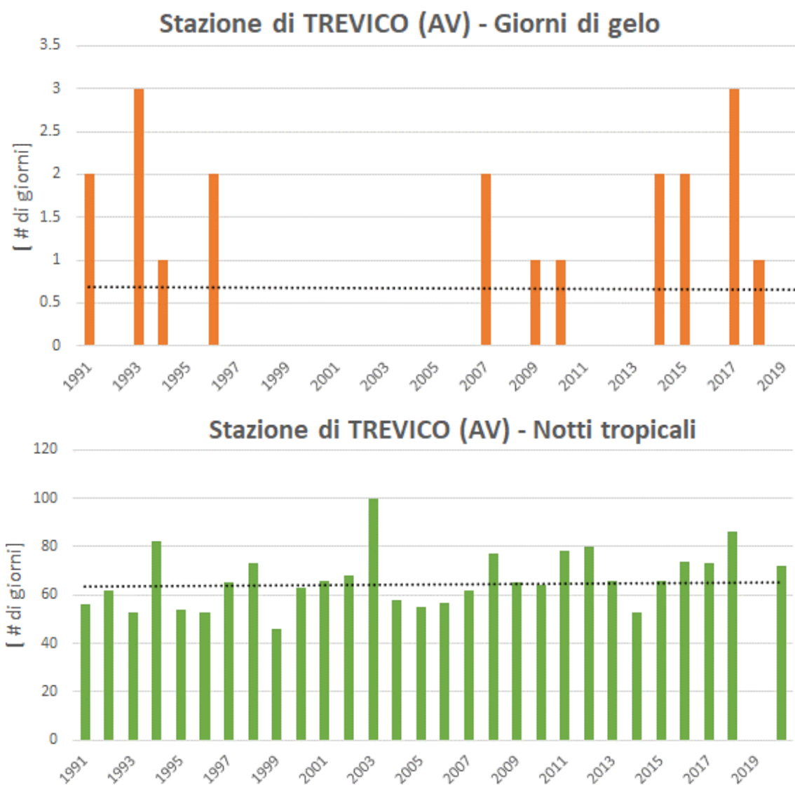
Figura 1-10: Giorni di gelo, notti tropicali e giorni estivi. Valori relativi alla stazione sinottica di Treviso (fonte: nostra elaborazione da dati SCIA)
