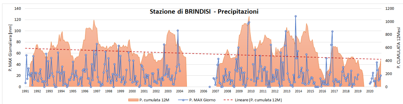
Figura 1-16: Precipitazione cumulata su 12 mesi e precipitazione massima giornaliera. Valori relativi alla stazione sinottica di Brindisi (fonte: nostra elaborazione su dati SCIA).
