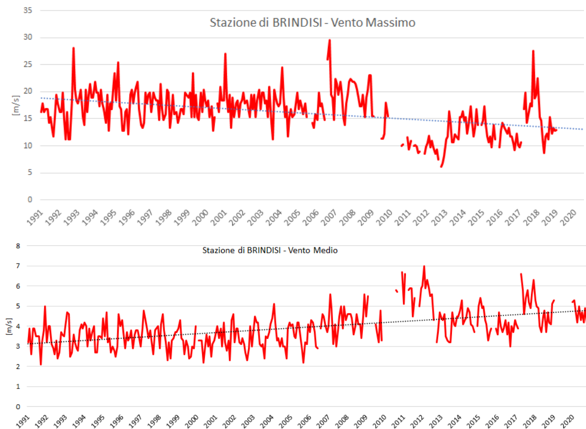
Figura 1-17: Venti massimi e venti medi. Valori relativi alla stazione sinottica di Brindisi (fonte: nostra elaborazione su dati SCIA).
