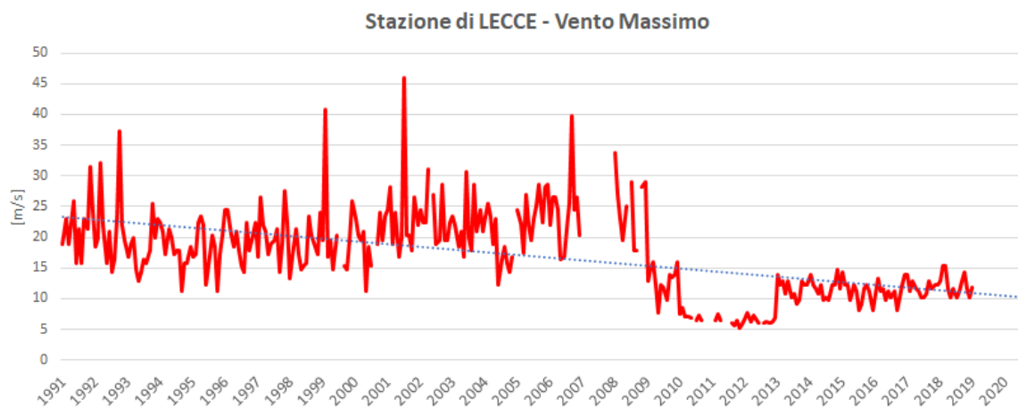
Figura 1-29: Venti massimi. Valori relativi alla stazione sinottica di Lecce (fonte: nostra elaborazione su dati SCIA).
