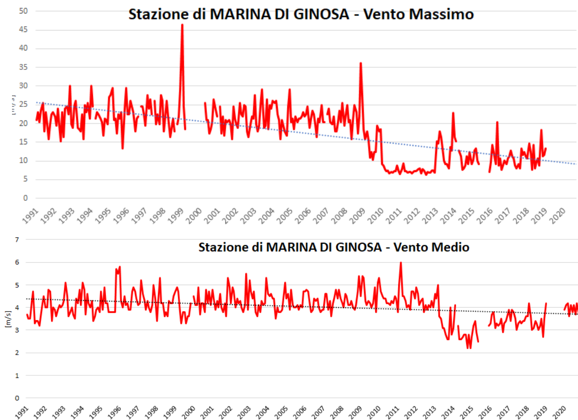
Figura 1-35: Venti massimi e venti medi. Valori relativi alla stazione sinottica di Marina di Ginosa (fonte: nostra elaborazione su dati SCIA).
