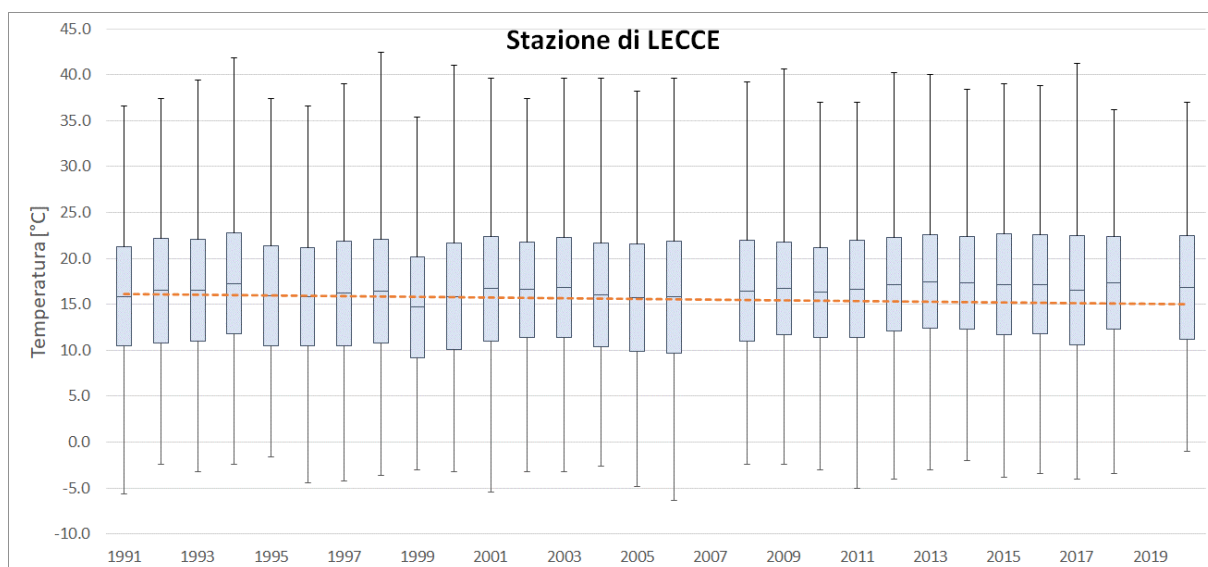
Figura 1-24: Andamento delle temperature annuali medie, minime e massime (medie mensili e assolute) per il trentennio 1991 - 2020 misurate nella stazione sinottica di Lecce (fonte: nostra elaborazione su dati SCIA)
