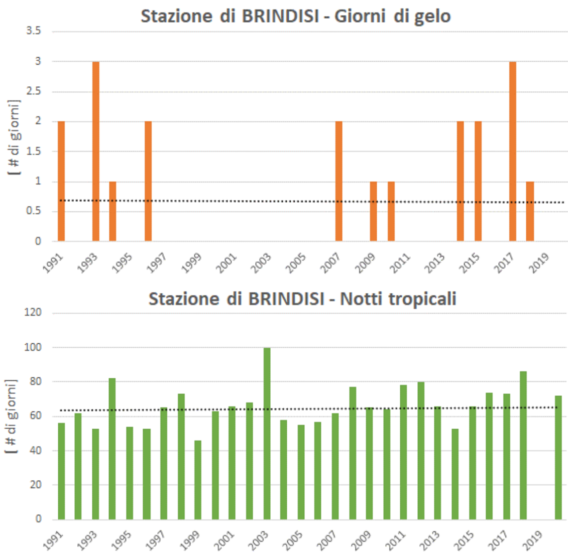
Figura 1-15: Giorni di gelo, notti tropicali e giorni estivi. Valori relativi alla stazione sinottica di Brindisi (fonte: nostra elaborazione da dati SCIA)
