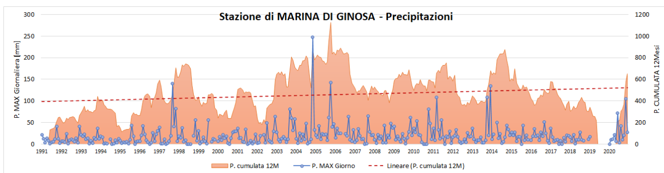
Figura 1-34: Precipitazione cumulata su 12 mesi e precipitazione massima giornaliera. Valori relativi alla stazione sinottica di Marina di Ginosa (fonte: nostra elaborazione su dati SCIA).
