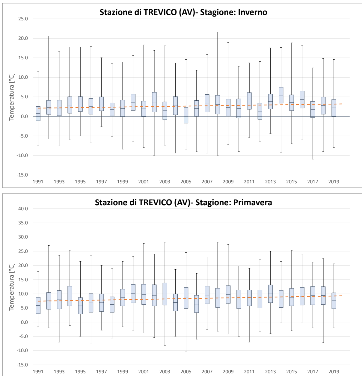
Figura 1-8: Andamento delle temperature stagionali medie, minime e massime (medie e assolute) per il periodo 1991- 2020 misurate nella stazione sinottica di Treviso (fonte: nostra elaborazione su dati SCIA)
