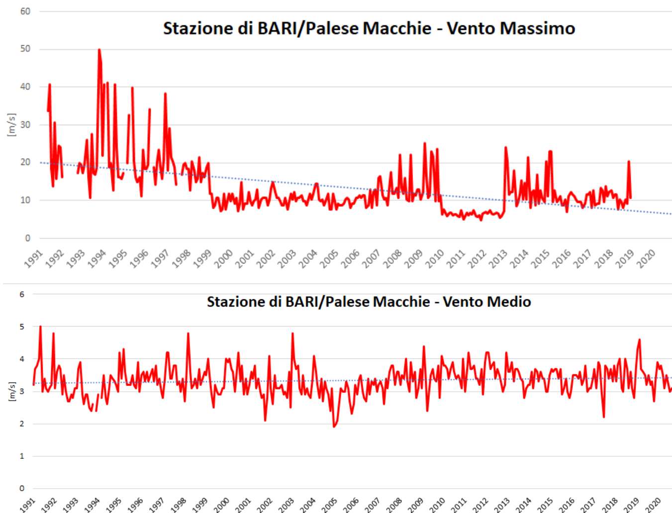
Figura 1-6: Venti massimi e venti medi. Valori relativi alla stazione sinottica di Bari/Palese Macchie (fonte: nostra elaborazione su dati SCIA).
